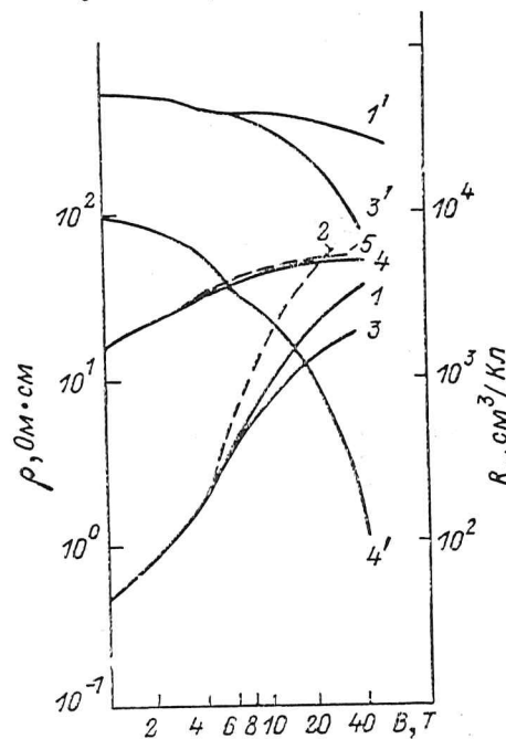
Рис. 3. Магнитолевые зависимости \rho_{\perp} (1—5) и R_H (1', 3', 4') для исходного образца (1—3, 1', 3'), для индентированного образца через t \sim 10^6 с (4, 4', 5).
